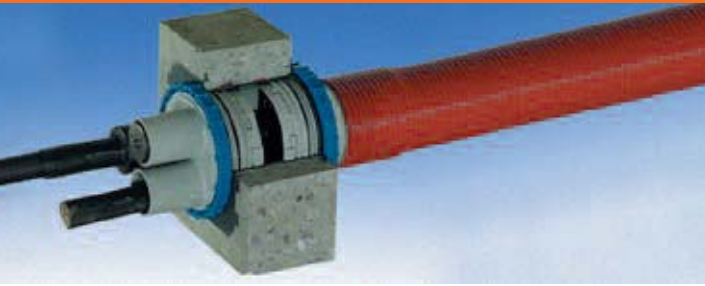
Druckwassersichere Waddurchführung
