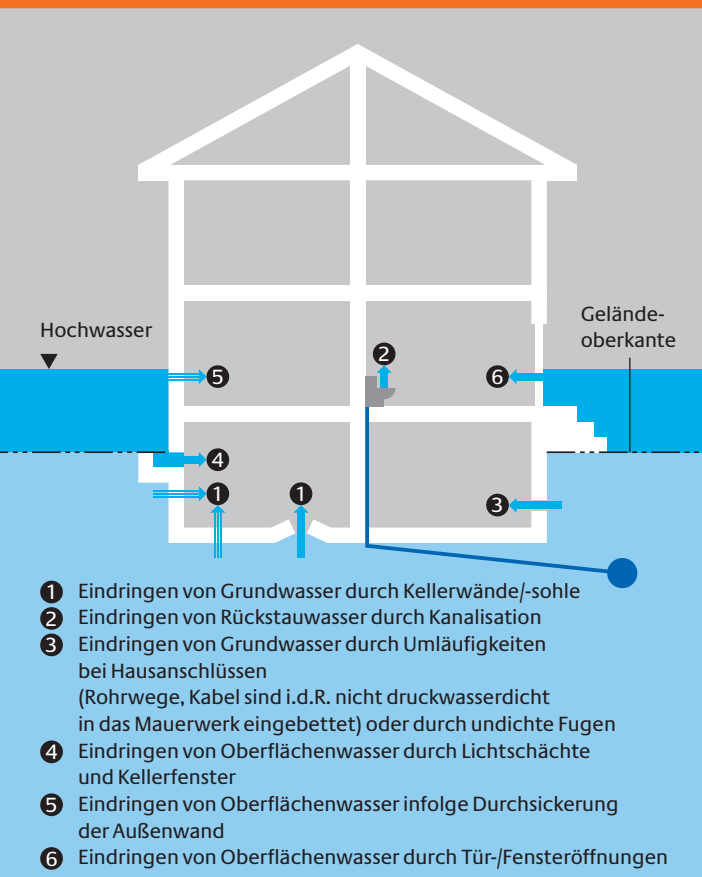
Wassereintrittsmöglichkeiten bei Gebäuden
